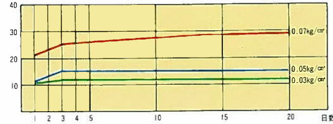
クリーフ23℃ 歪%
